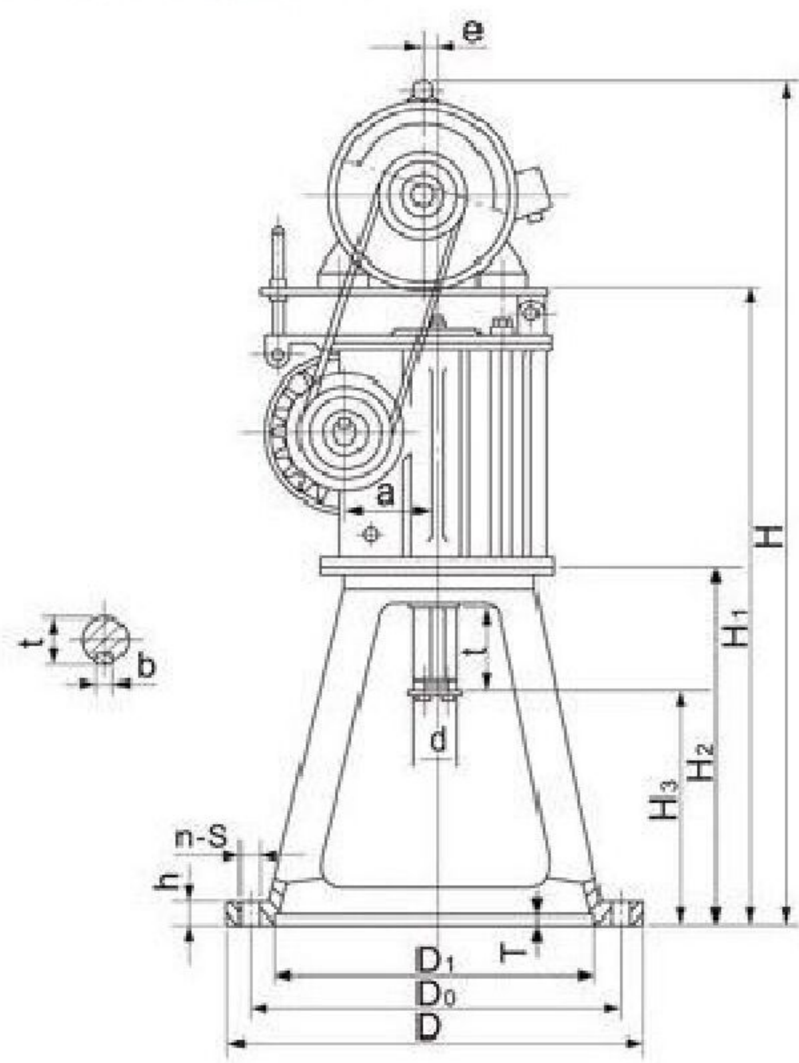
LCW系列外形安装尺寸
