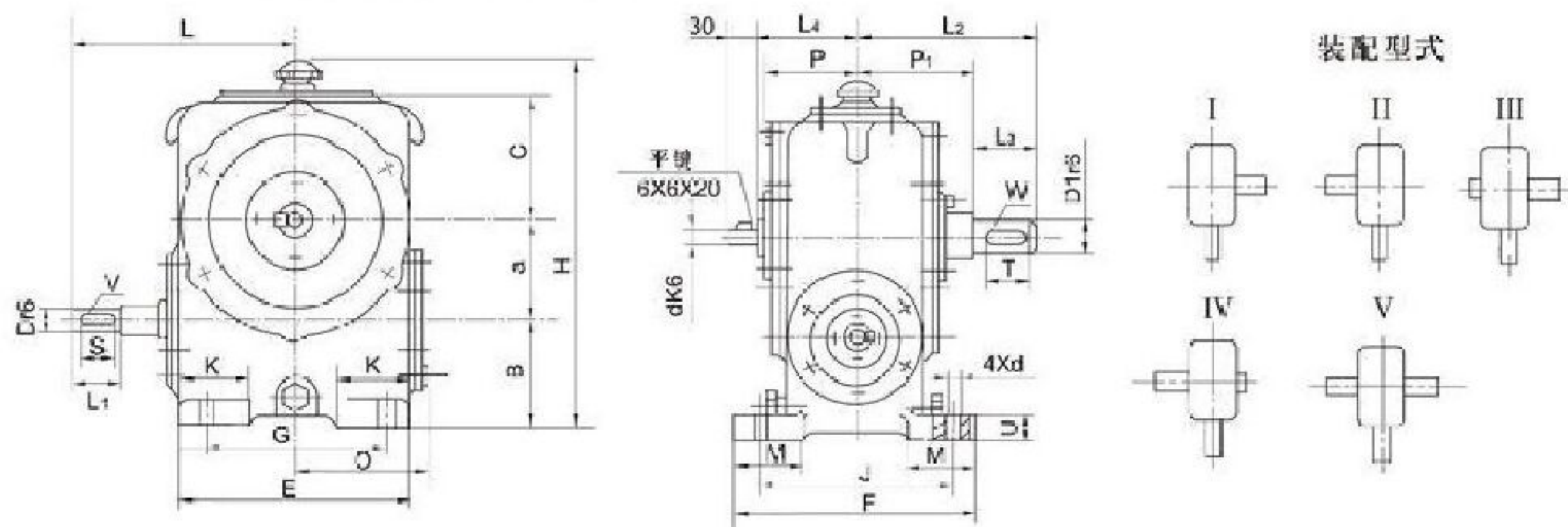
WD80-120型减速器外形尺寸及装配型式
