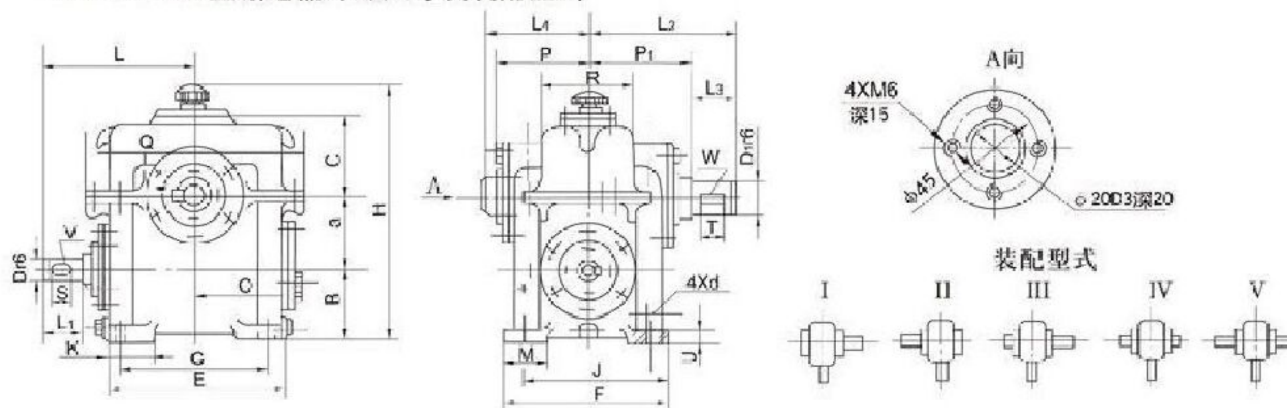
WD150-360型减速器外形尺寸及装配型式
